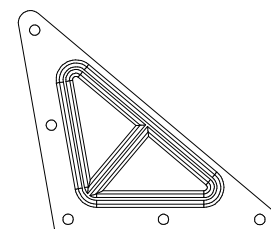
(2) DO - BRAZO AMARILLO DEL COLUMPIO TIPO PLANEADOR DEL CAPITÁN - A100026
